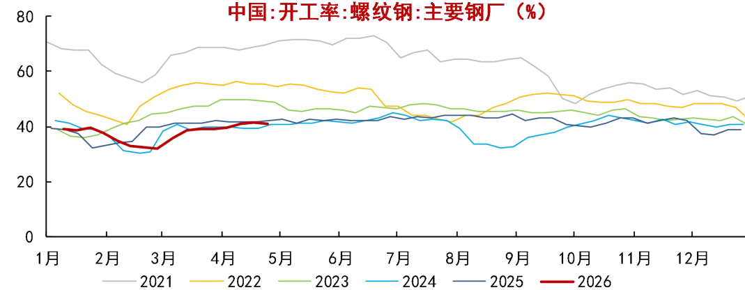
中国:开工率:螺纹钢:主要钢厂 (%)
